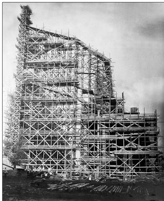
Строительство главного корпуса КазГРЭС (ТЭЦ-1). Казань. 1930 г. ИМ РТ
